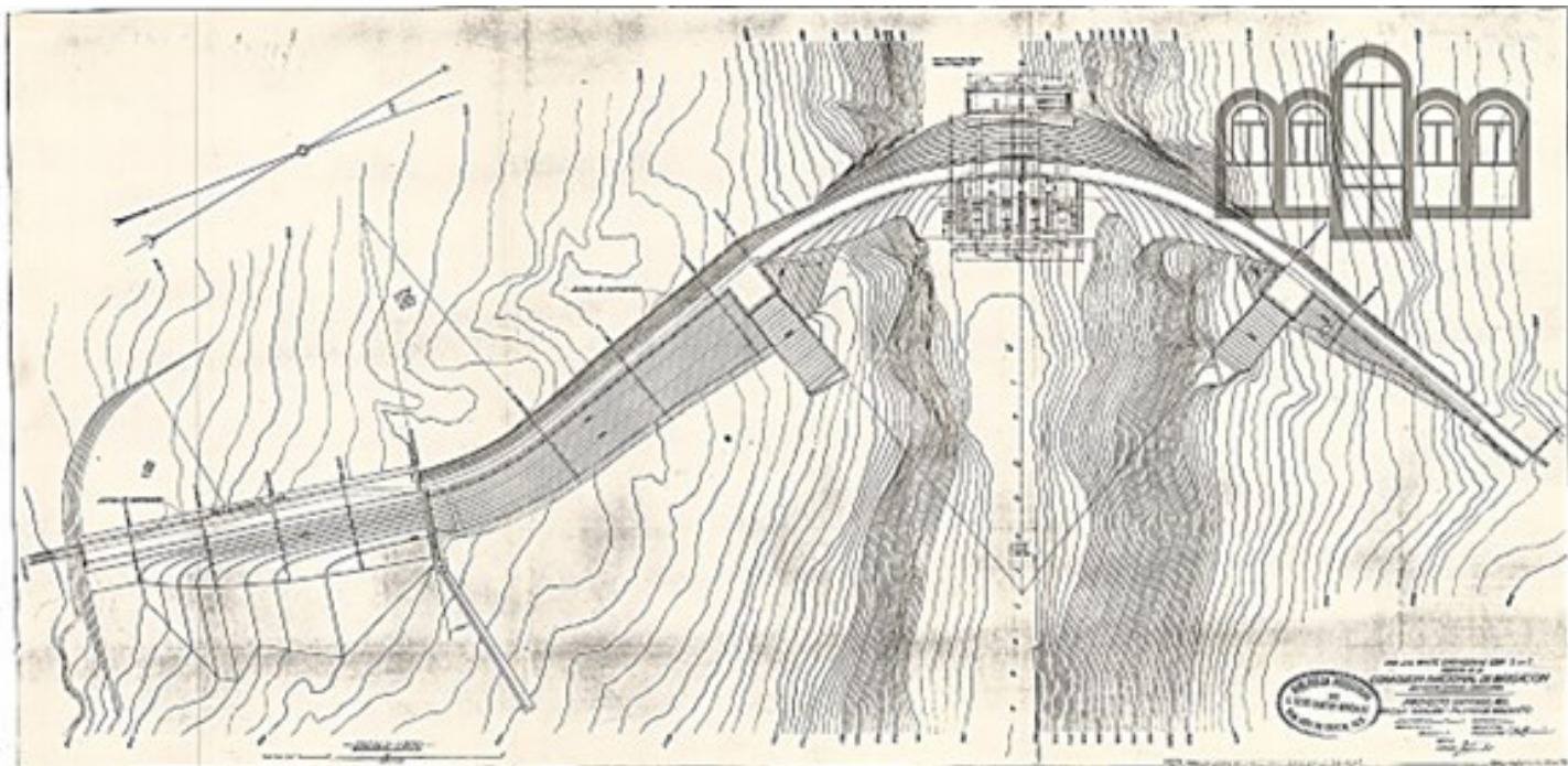
Plano de la cortina de la presa “Presidente Plutarco Elías Calles”, San José de Gracia, Ags. Fuente: el autor.
